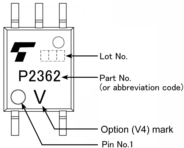
Fig. 16.4 Marking Example(Note)
